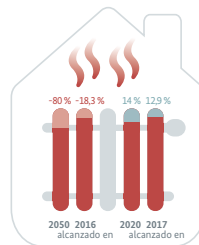
Demanda de energía primaria en edificios (frente a 2008)
