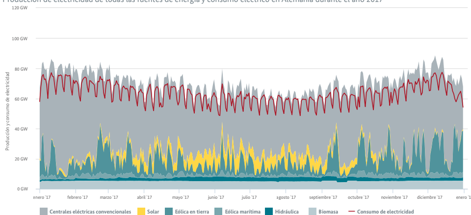
Producción de electricidad de todas las fuentes de energía y consumo eléctrico en Alemania durante el año 2017
